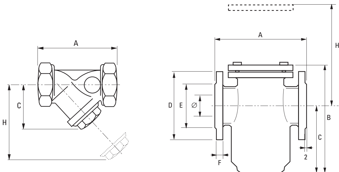
Filtre "Y"
