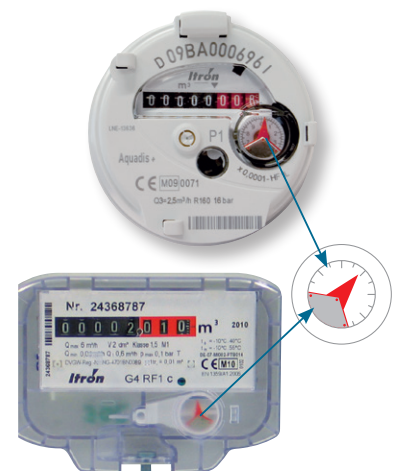
Itron Wasserzähler Zählwerk mit Cyble Target
